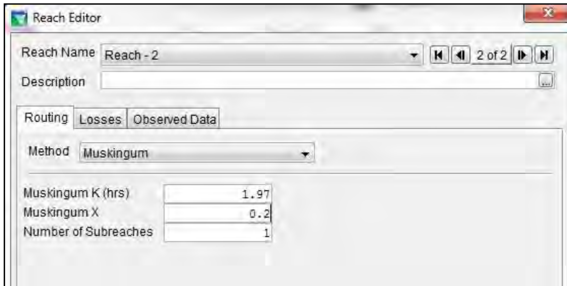
Figure 5-3 Reach Parameter
